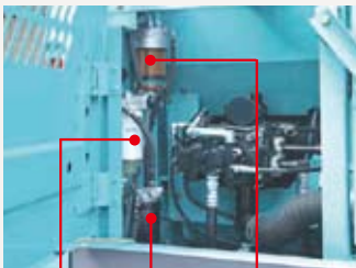
Filtro principal de combustible Pre-filtro de combustible (con separador de agua)
